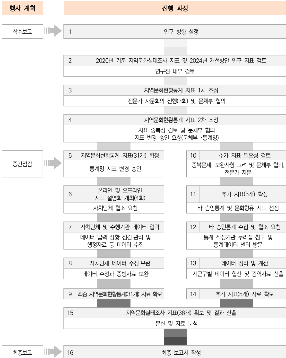
[그림 1-3-1] 연구흐름도
